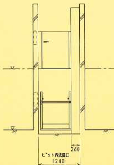
■ 升降路断面图（正面）
