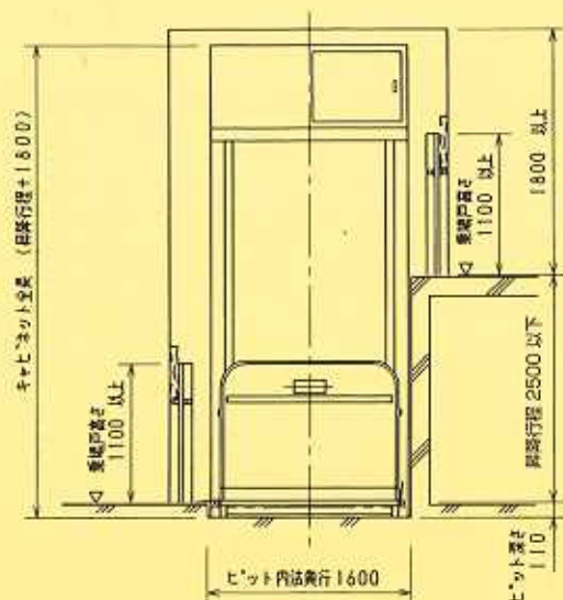
■昇降路断面図（側面）
