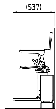
「いす」を広げたとき
