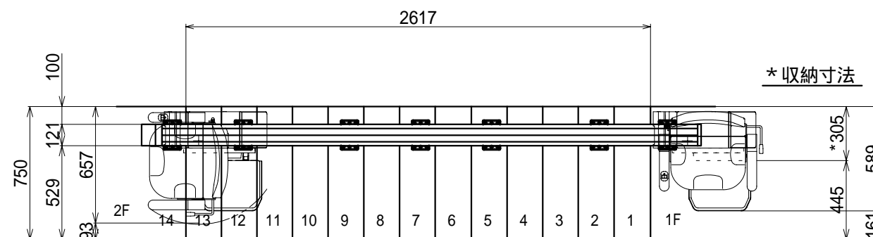
(階段平面図)
