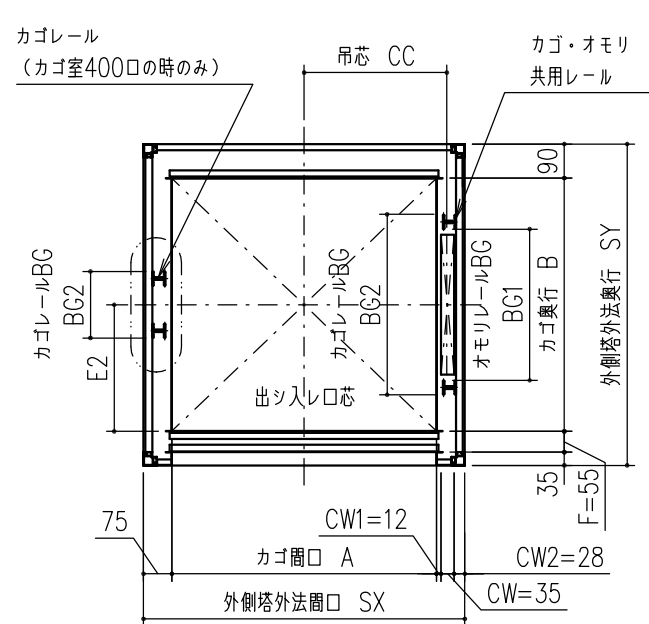
RU-D 升降路平面図
