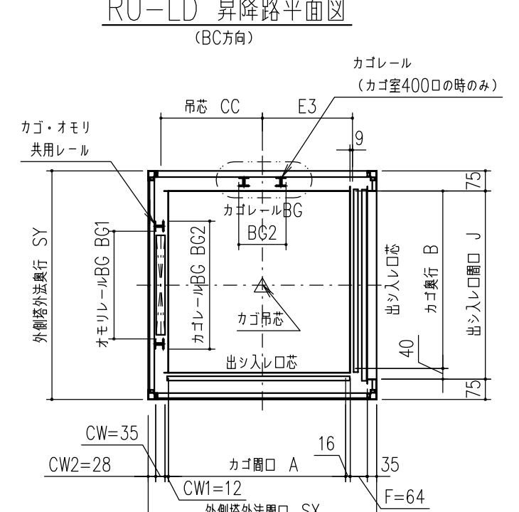
RU-LD 昇降路平面図
