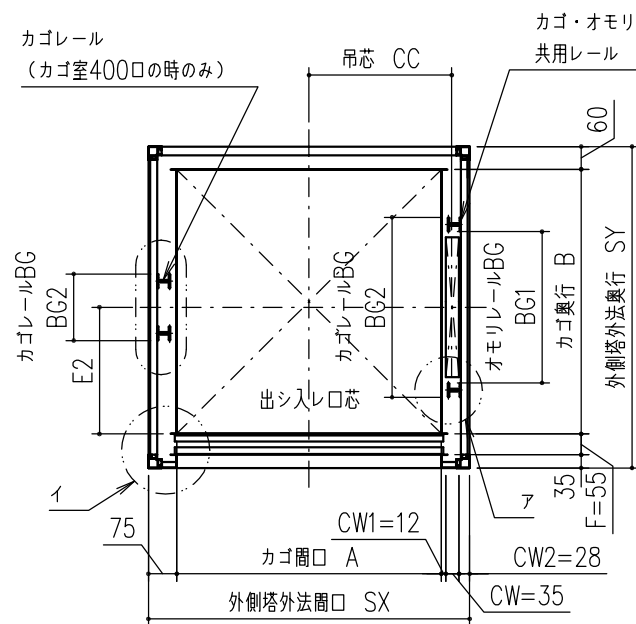
RU-S 升降路平面図
