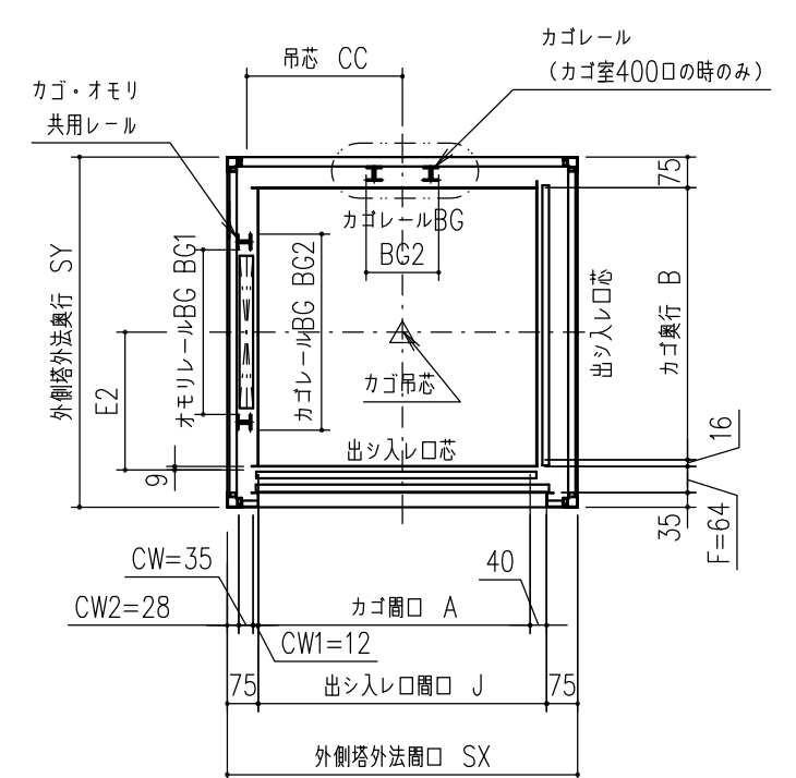
RU-LD 昇降路平面図
