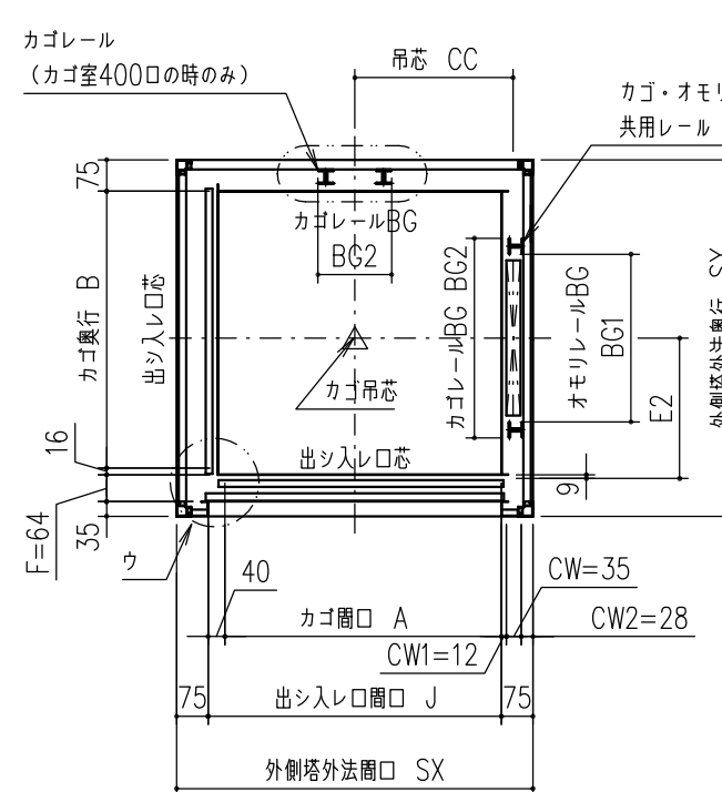
RU-LD 昇降路平面図
