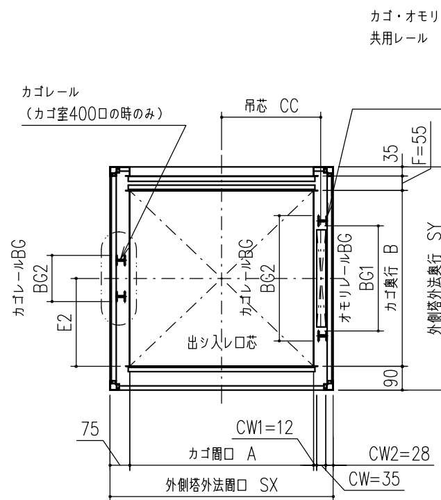
RU-D 升降路平面図
