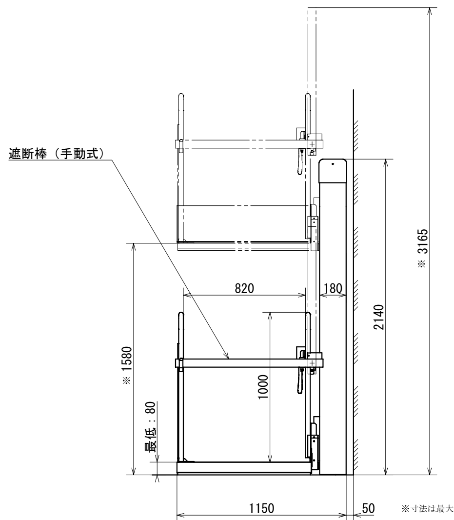
全体構造据付図 (DA-150Ad)
