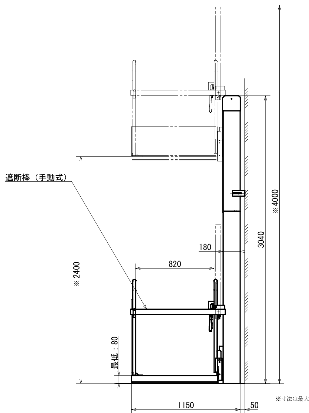
全体構造据付図 (DA-240Ad)
